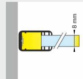
MIKRO-LINE12 Glass mounting Montaż na szybie
