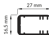
J J slide cover klosz J wsuwany
